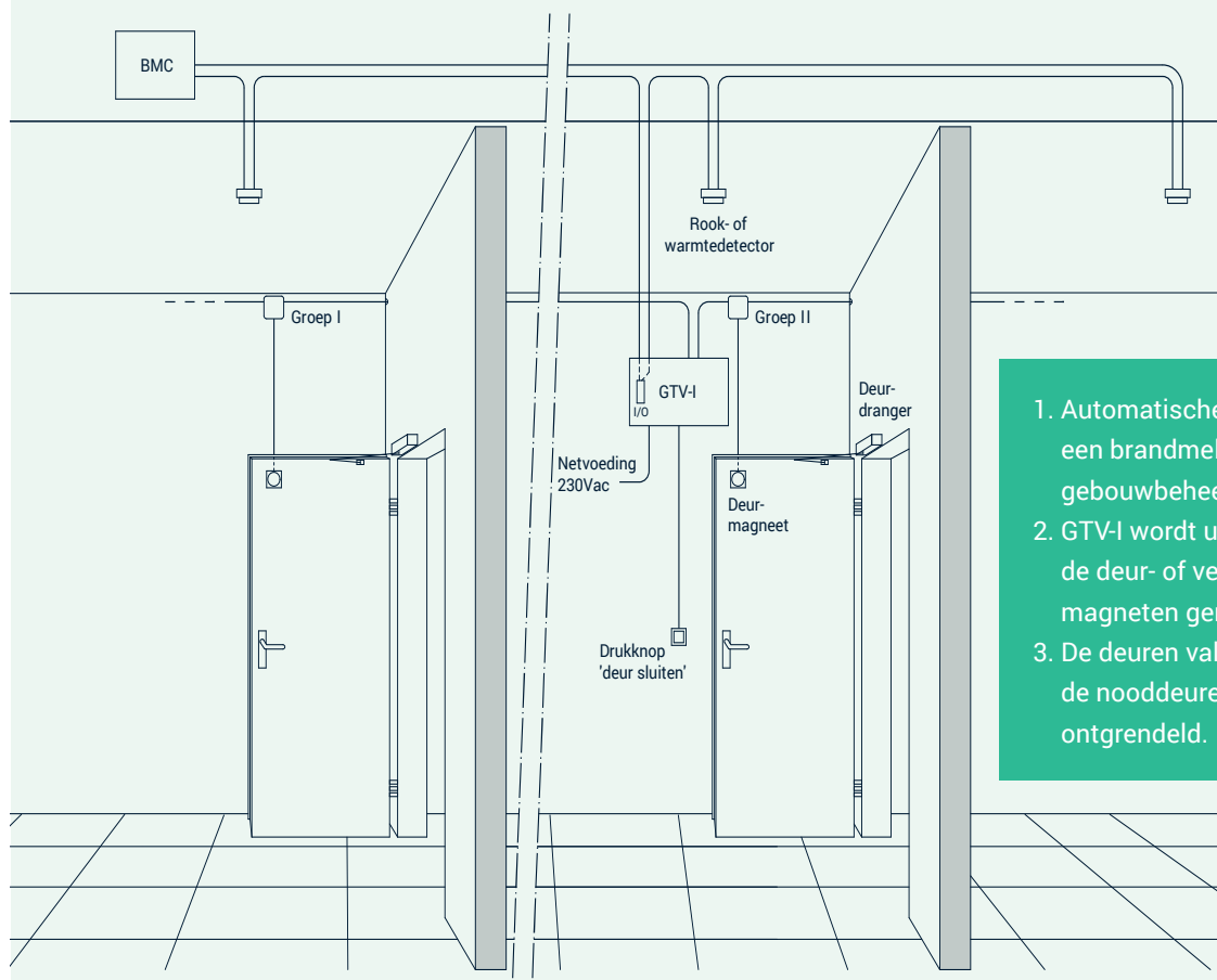
Principe deur ontgrendelsystemen met GTV-voedingen
